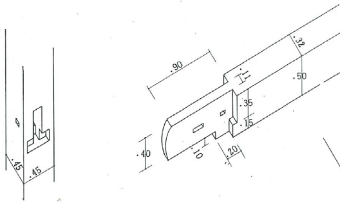
8 身舎東側梁行梁仕口
