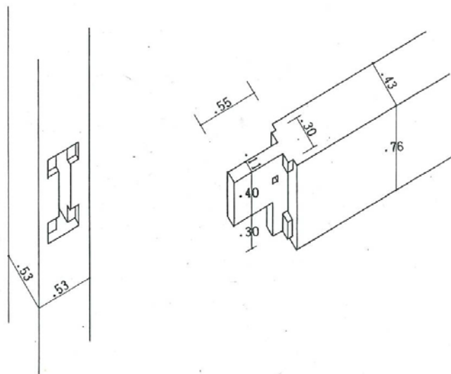
10 なかのま・おくのま境指物仕口
