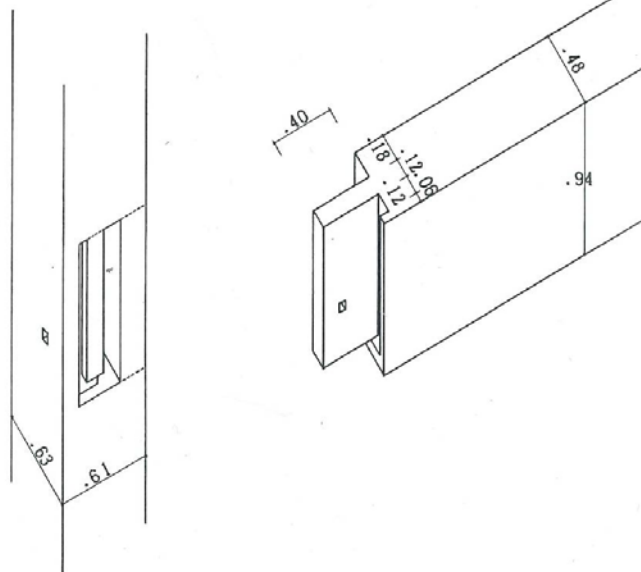
9 にわ・なかのま境指物仕口
