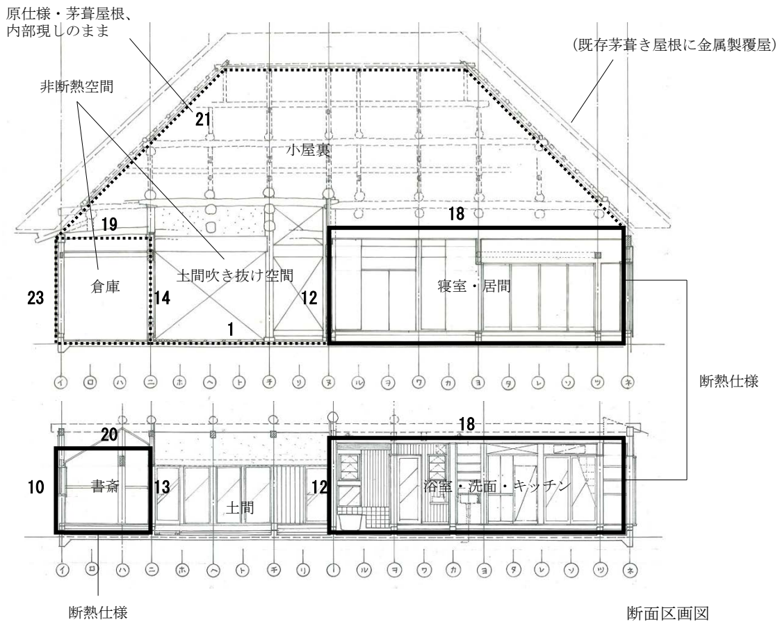
《用途と断熱仕様区画》
